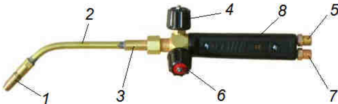
Рис.1 Горелка Г2; Г2У с наконечником ДЖЕТ 000 100 100-(01...11)
